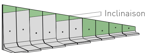
Éléments de hauteur différente sur fondation continue et avec bord supérieur incliné.
